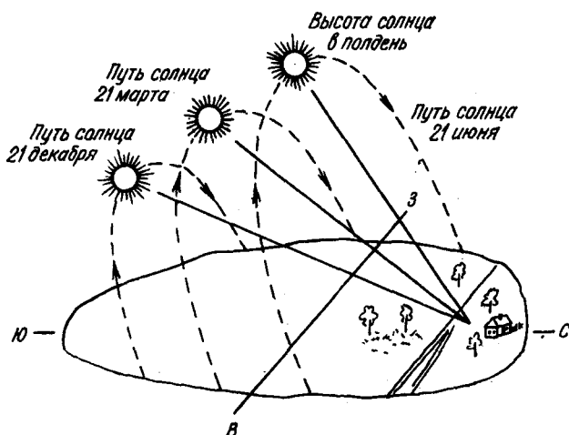
Рис. 3. Видимое движение Солнца в разные сезоны года
