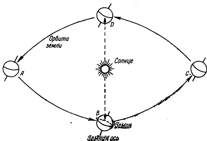
Рис. 2. Орбита Земли
