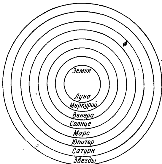
Рис. 5. Расположение планет
