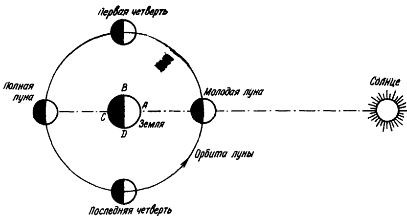
Рис. 1. Лунный цикл
