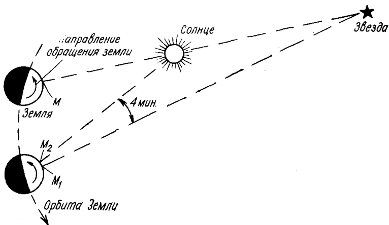
Рис. 4. Солнечный и звездный день
